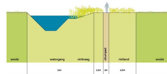
profiel A-A'
