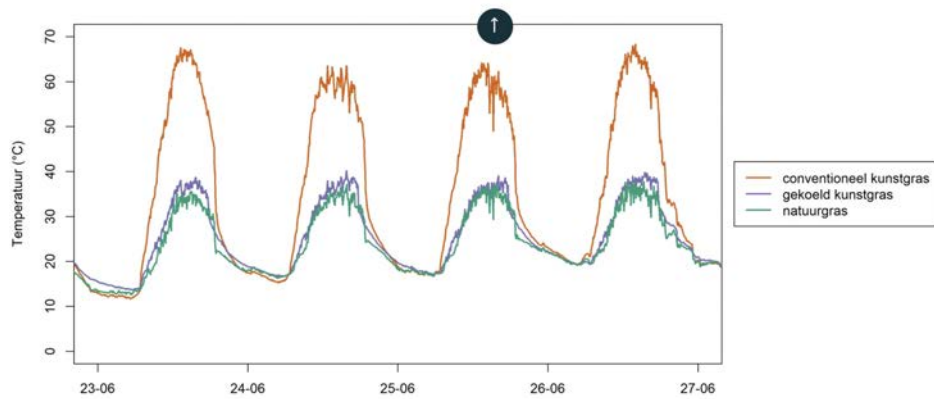
Oppervlaktetemperatuur gemeten op de proefvlakken voor de verschillende systemen voor de periode 23 juni tot 27 juni 2020
