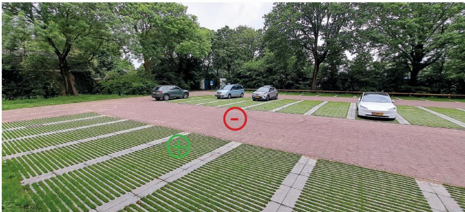
Beheer uitgangspunt: rijloper in dichte verharding
